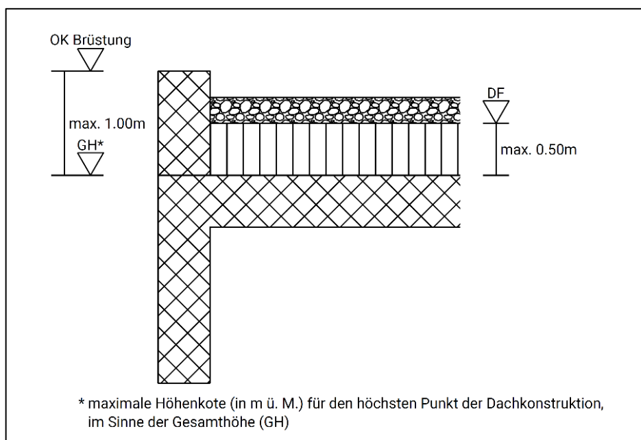
Abb. 7: Skizze Messweise der Gesamthöhe (GH), Dachfläche (DF) und Brüstung (OK Br)
